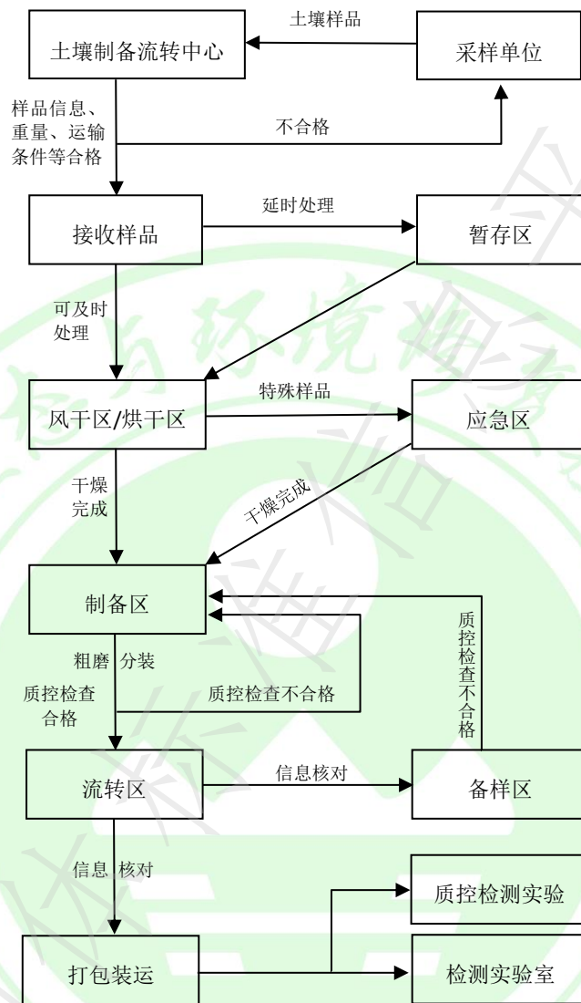
图1 运行流程图
